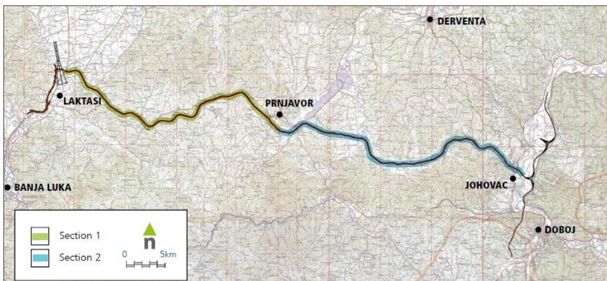
Slika 2.2: Dionica 2 Prnjavor - Doboј
